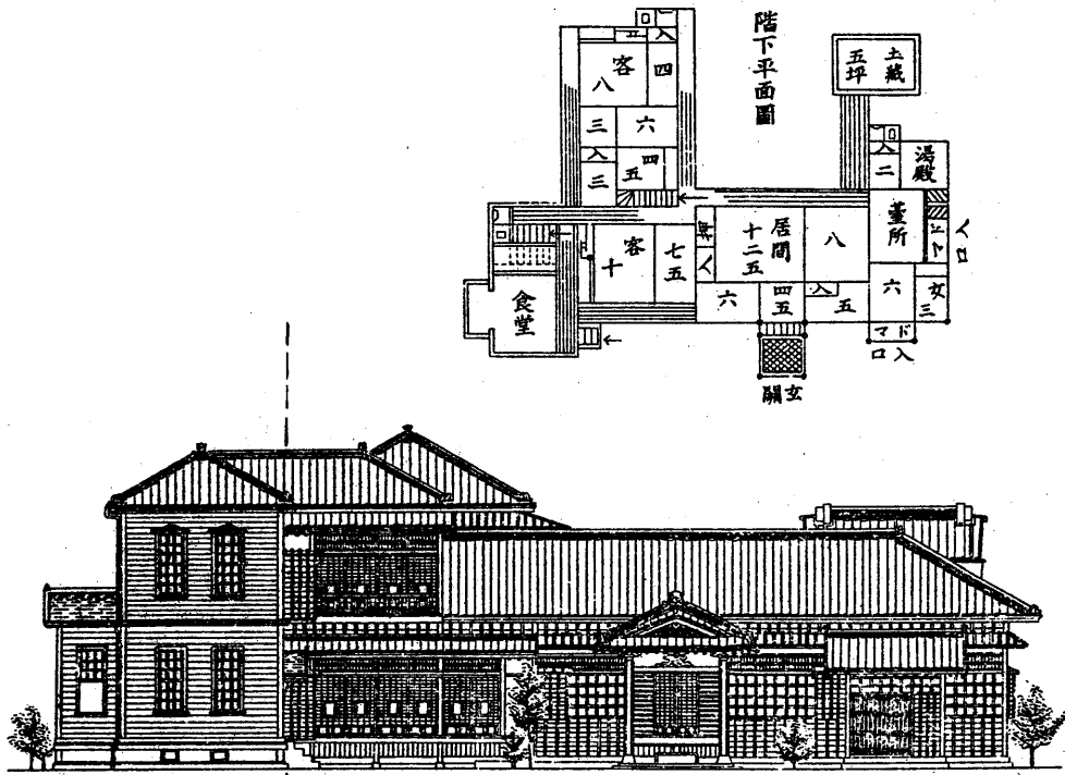
図4 明治後期中流住宅「和洋折衷住宅」の正面図と階下平面図
