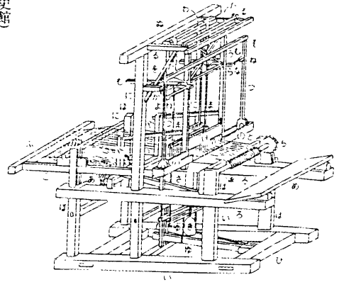
日本の力織機（1900年頃）—特許第1195号（織機）
