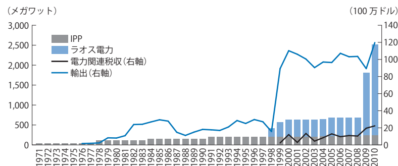
図2 ラオスにおける所有形態別総発電能力の推移
