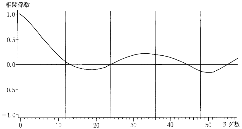
第4図 CDIの自己相関(コログラム)
